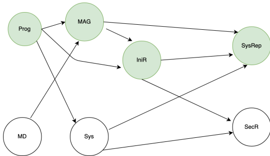
Figure 104 – Au moins 4 semestres sont nécessaires pour obtenir ce master. Cela peut se calculer par l'algorithme Vertex-rank-longest-paths(G,I,s) qui permet de calculer le plus long chemin (PLC) du premier au dernier niveau dans un graphe par niveaux.
