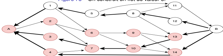
Figure 78 – On construit un flot de valeur 3.
