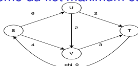
Figure 116 – Un graphe G = (V, E, c) avec des capacités c_e, e \in E .
