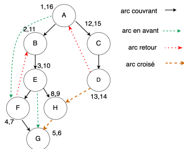
Figure 39 – L'arborescence de l'appel DFS(G, A) .
