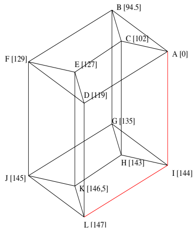
Figure 113 – Les points extrêmes du domaine (il y en a douze) et les valeurs de la fonction objectif correspondantes. Le parcours de l'algorithme de simplexe est visualisé en rouge. Deux itérations suffisent pour trouver l'optimum.
