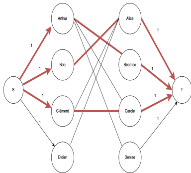
Figure 122 – La valeur du flot maximum vaut aussi 3.
